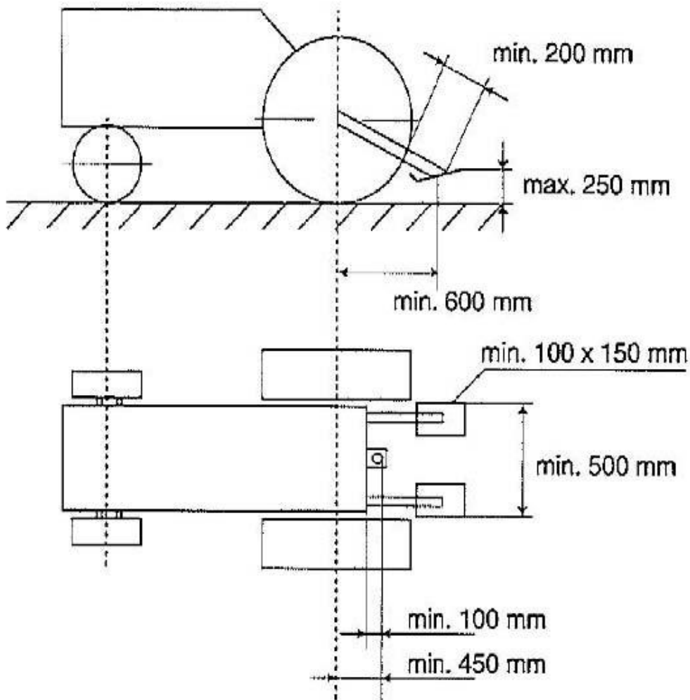
Figuur 31: constructie/maatvoering steigerbegrenzer
