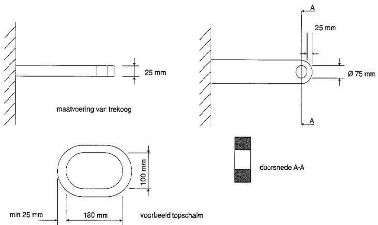
Figuur 32: maatvoering trekoog en topschalm
